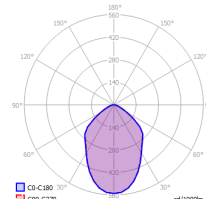
EMLB z odbłyśnikiem symetrycznym
