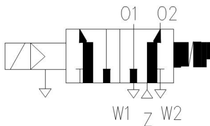
Rozdzielacz FERPI-5/2-1-S
