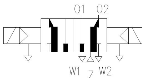
Rozdzielacz FERPI-5/2-1
